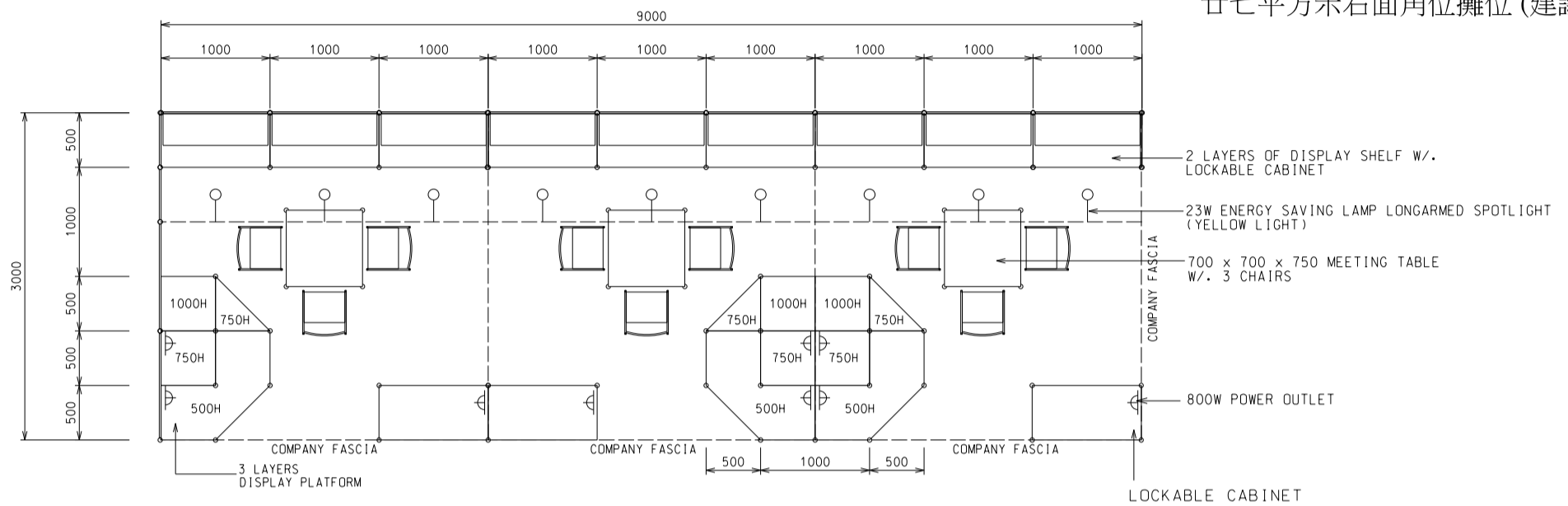
PLAN 9M(W) X 3M(D) X 2.5M(H) RIGHT CORNER BOOTH B
